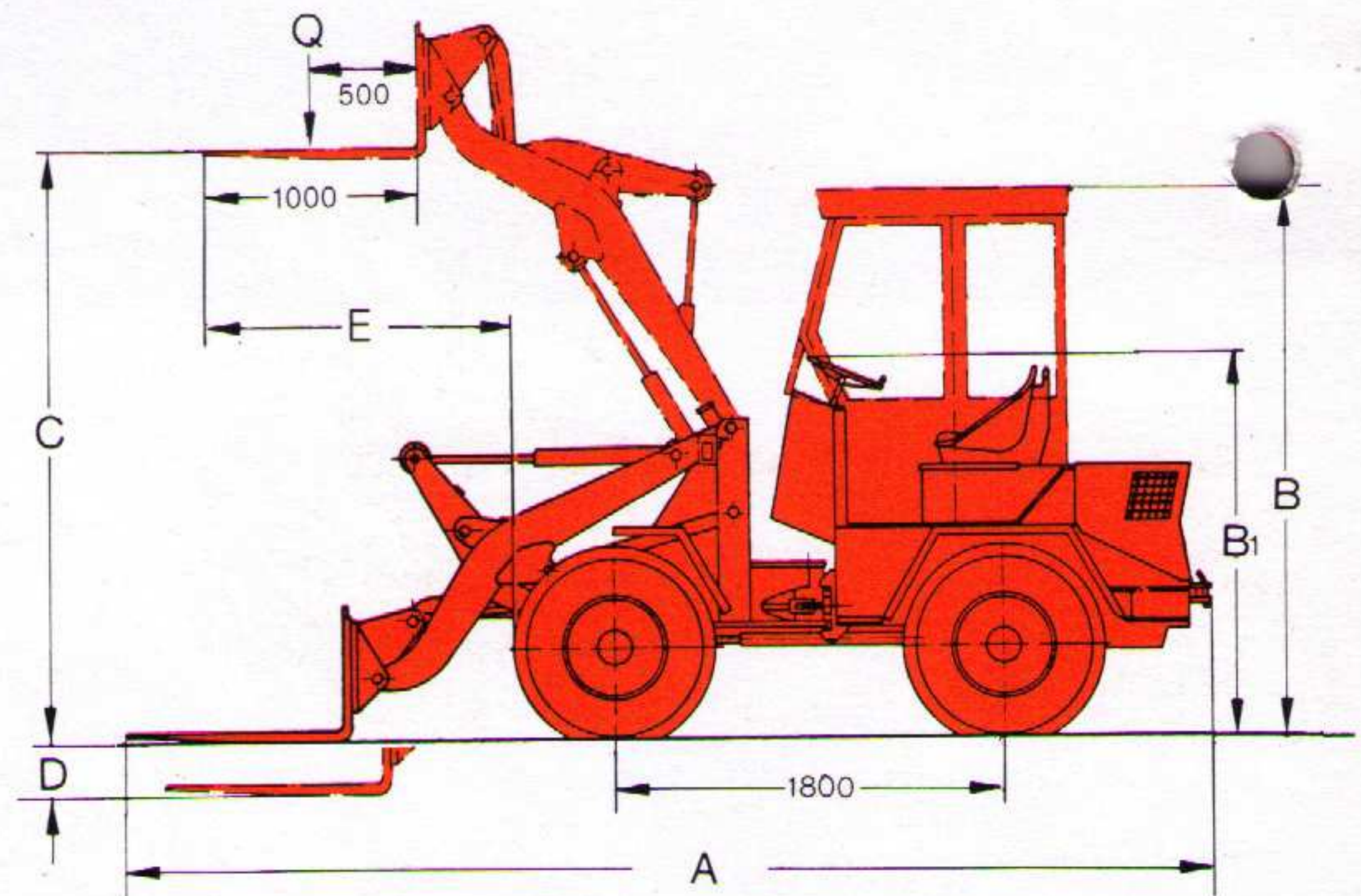
Technische Angaben mit Palettengabel
