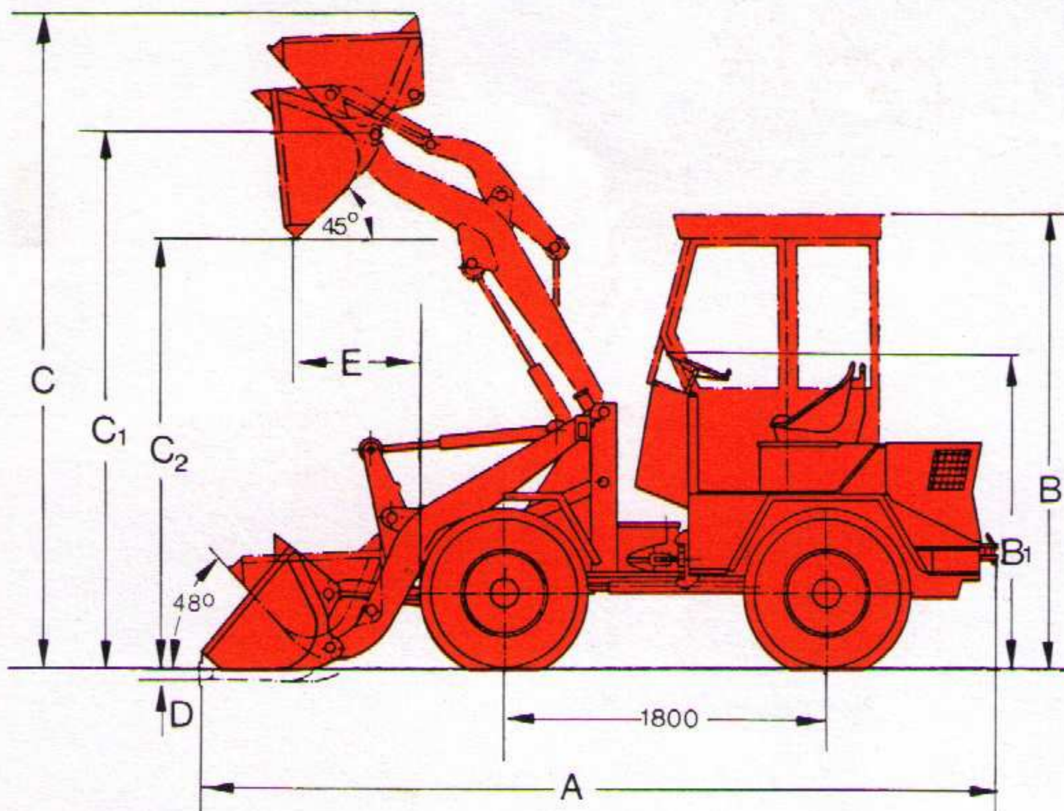
Technische Angaben mit Leichtgutschaufel
