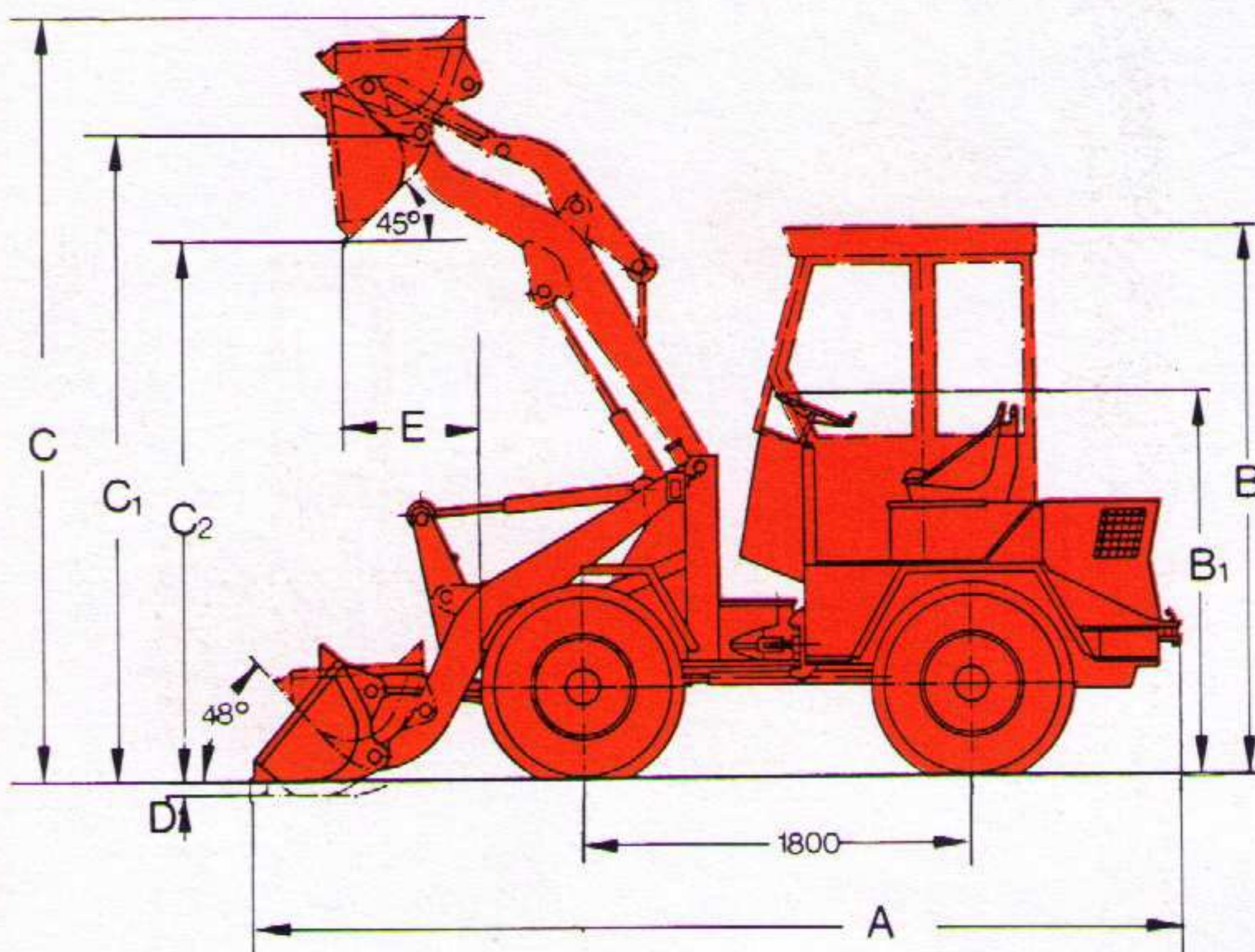
Technische Angaben mit Standardschaufel
