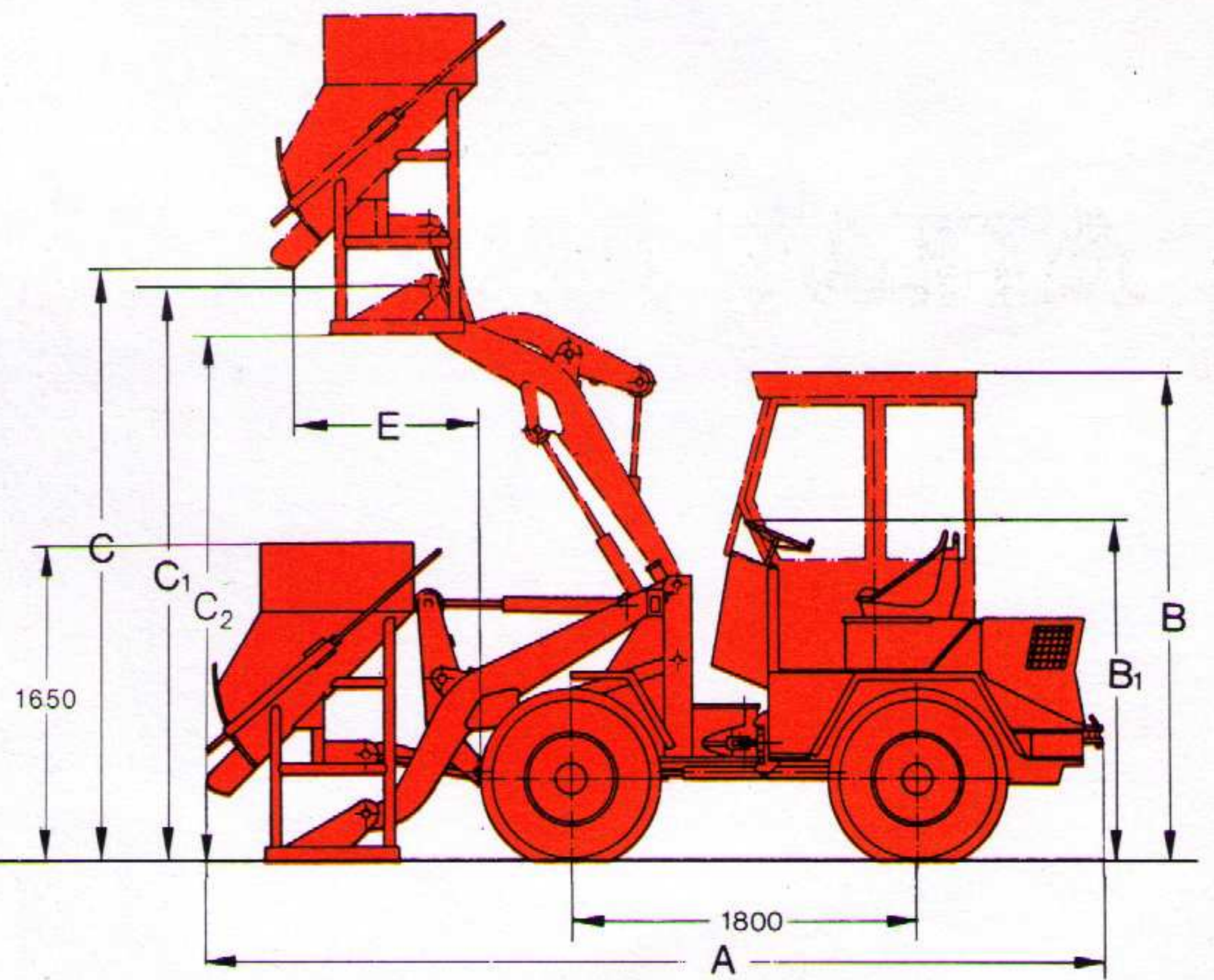
Technische Angaben mit Betonkübel
