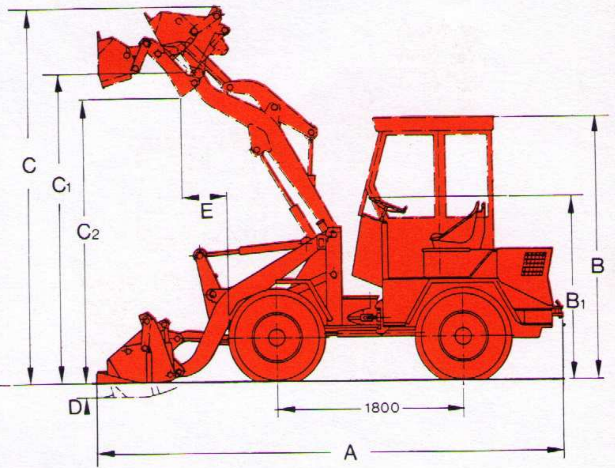
Technische Angaben mit Uni-Schaufel
