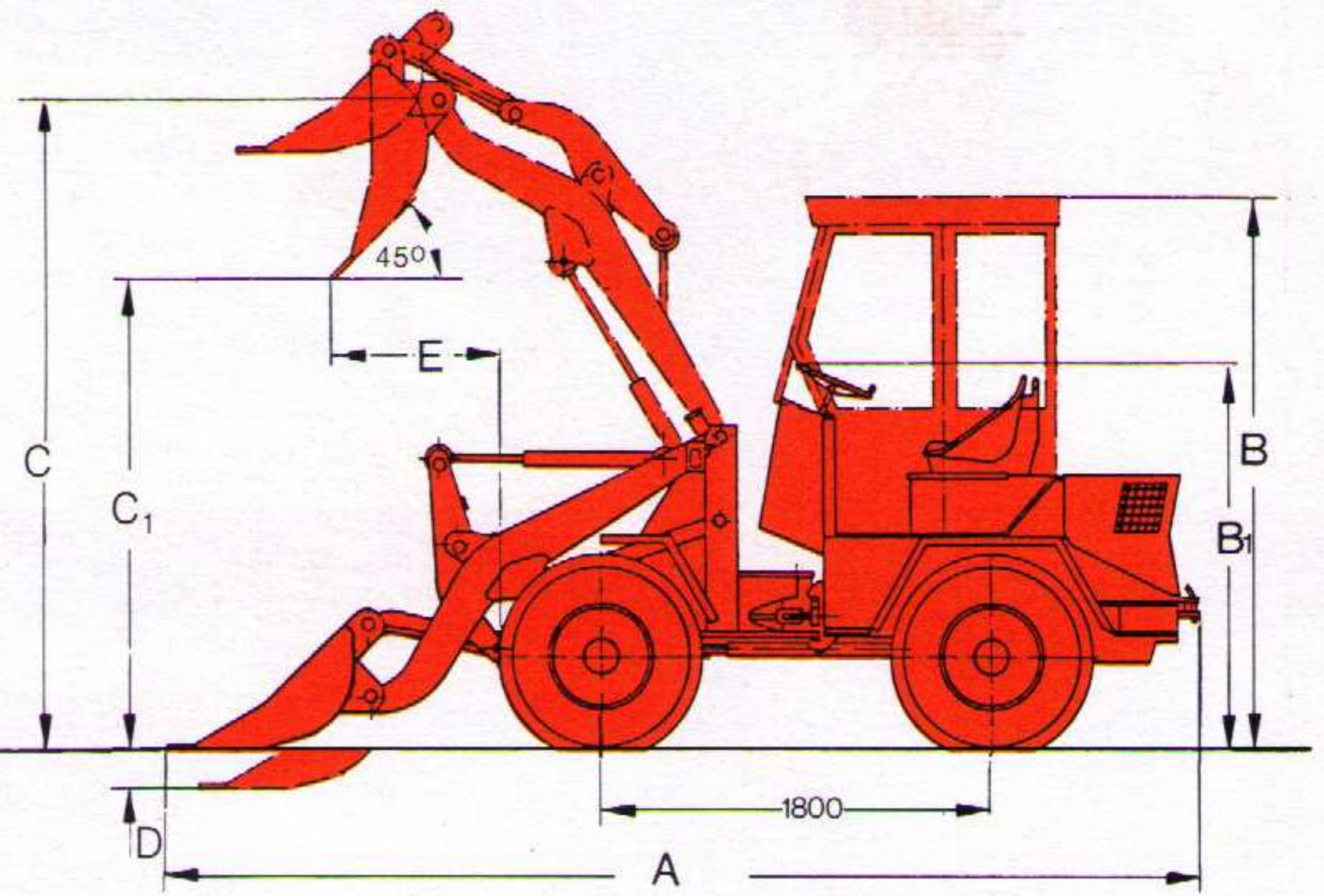
Technische Angaben mit Steingabel
