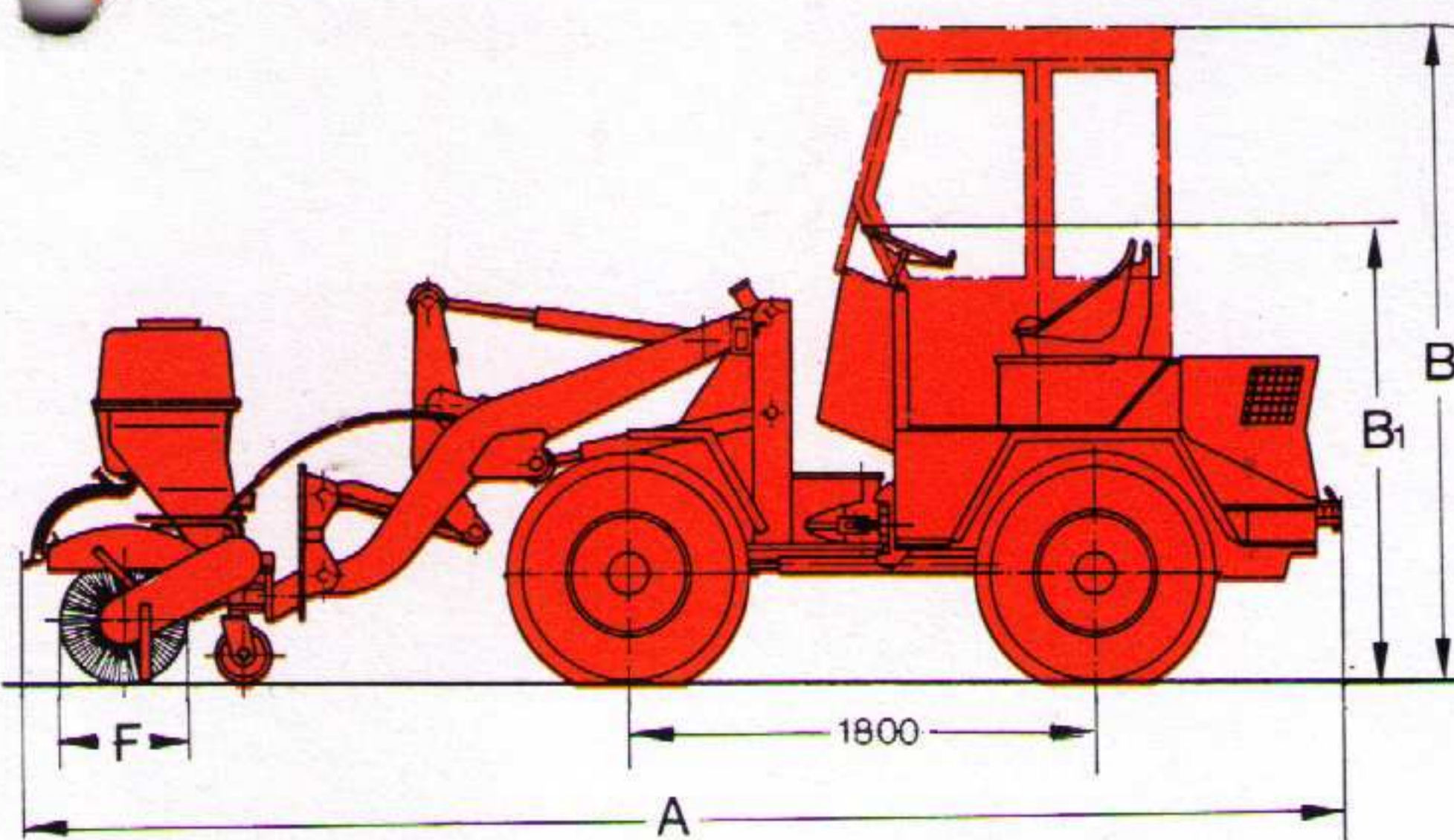
Technische Angaben mit Kehmaschine einschl. 200-l-Wasserbehälter
