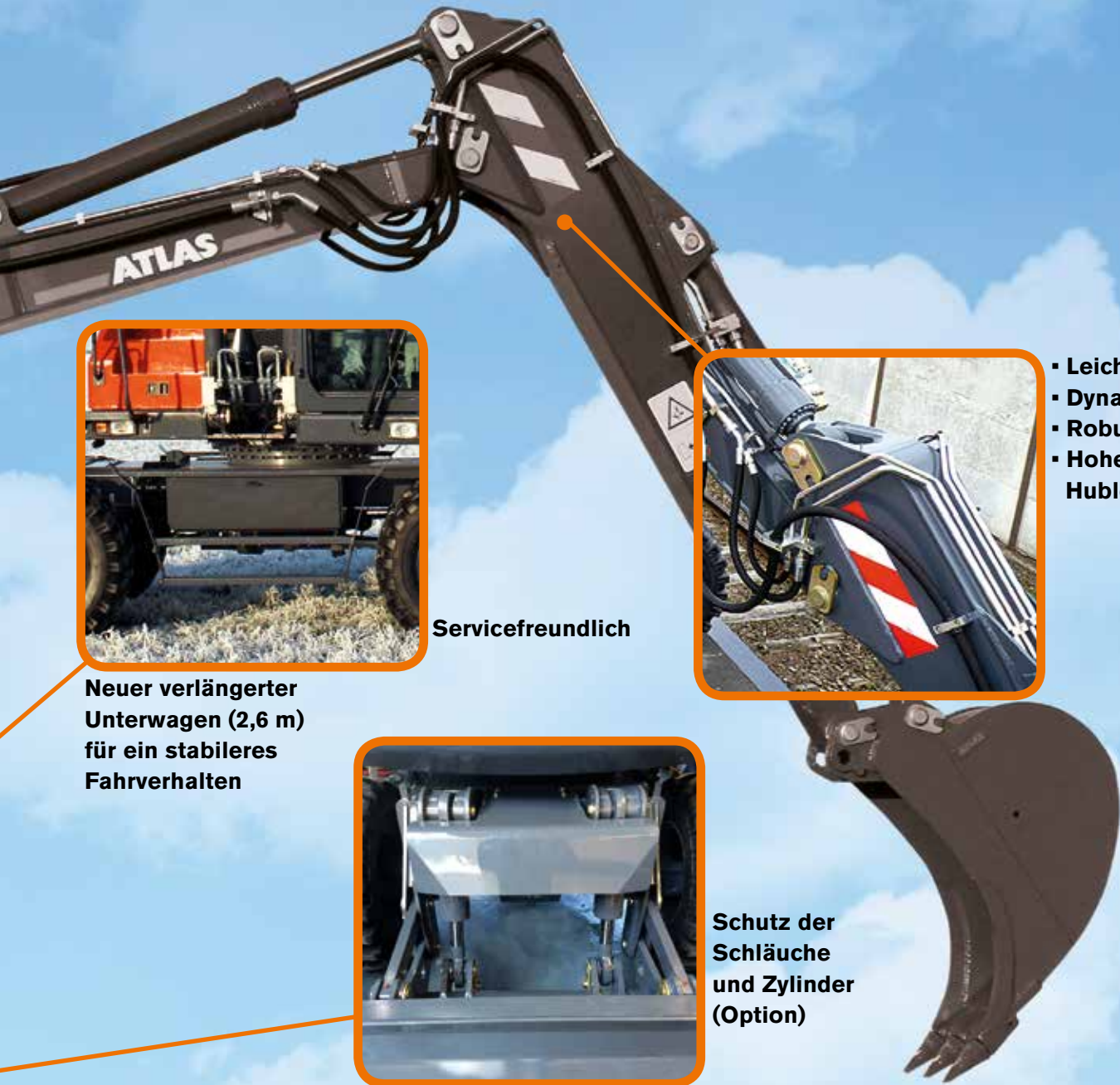
Bremsschlauchsicherung
