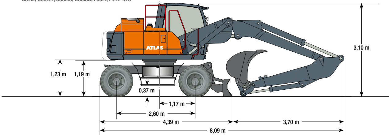
Transportstellung A67.2, C66.41, C66.46, D63.3A, F66.1, F412-415
